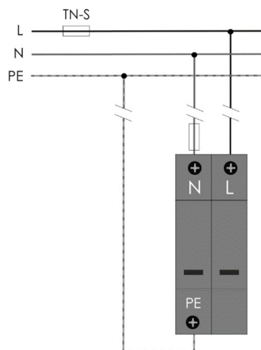
Koblingsskjema
