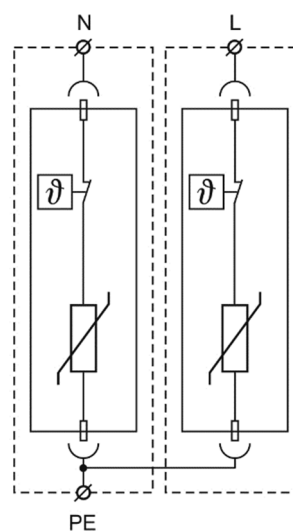
Internt koblings skjema
